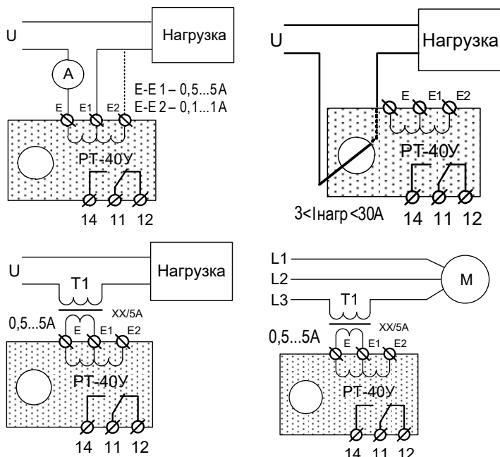
Рис. 1. Варианты схем подключения.
